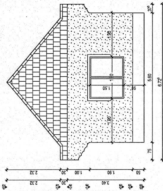
UTCAI HOMLOKZAT - MEGLÉVŐ ÁLLAPOT - M=1:50
